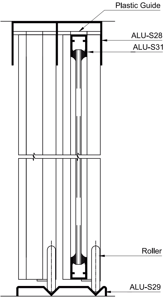
SECTION :- A-A
