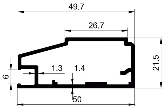
SECTION NO. - KCB-007 EST. WEIGHT - 0.563 KG./M.
