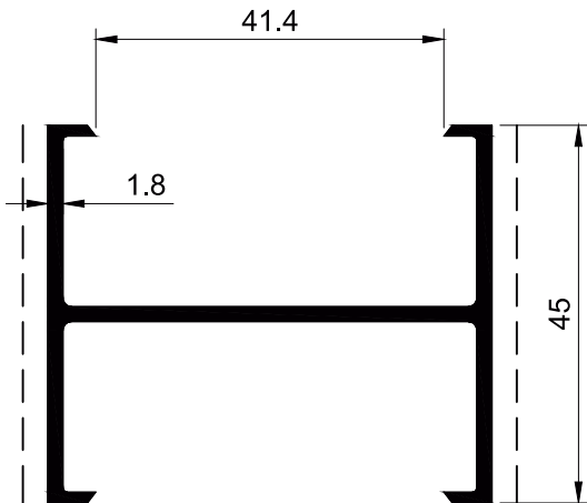
SECTION NO. - HDR-312 EST. WEIGHT - 1.428 KG./M.
