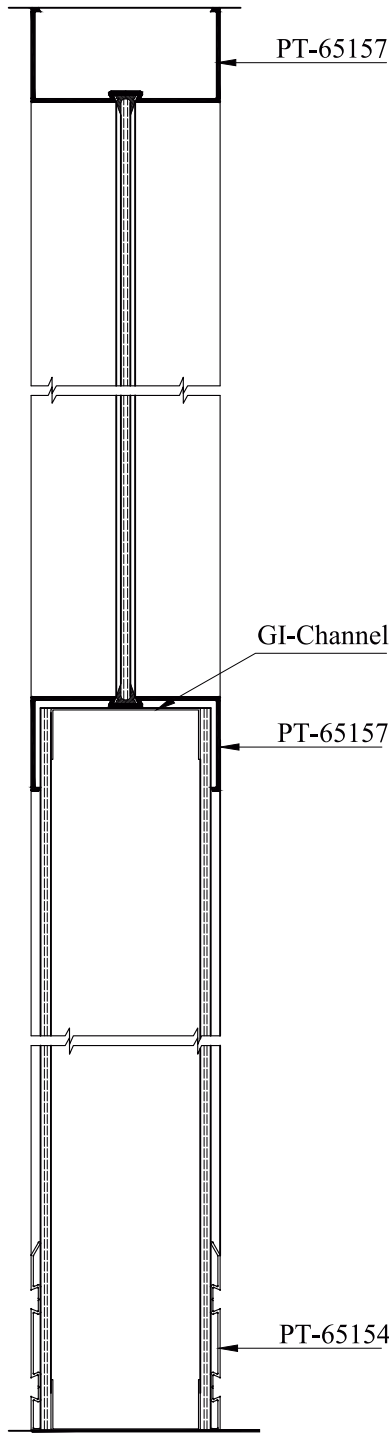
Section :- A-A
