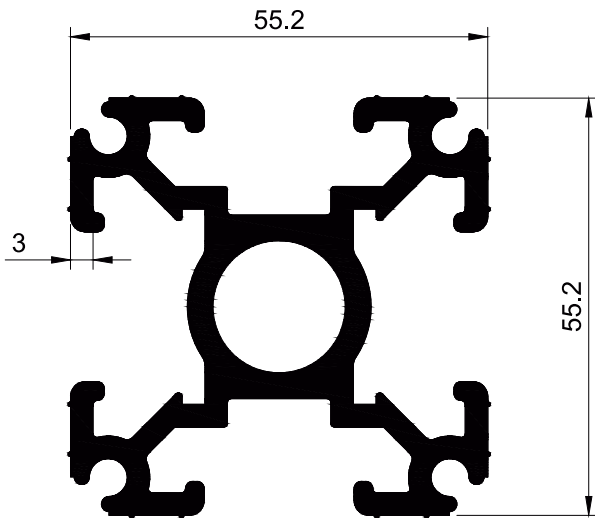
SECTION NO. - HDR-308 EST. WEIGHT - 2.440 KG./M.
