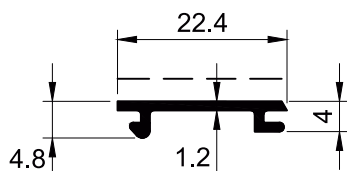
SECTION NO - LSD-1503
