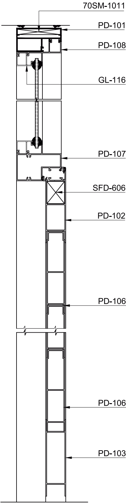
Section :- A-A
