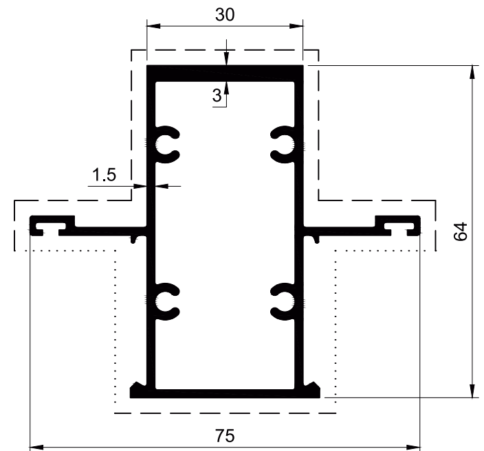
SECTION NO. - CA-1118 EST. WEIGHT - 1.280 KG./M.
