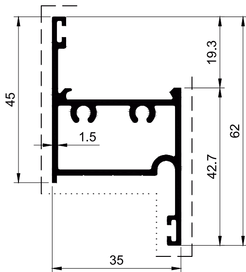
SECTION NO. - CA-2008 EST. WEIGHT - 0.766 KG./M.
