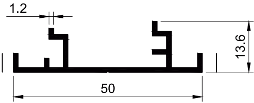
SECTION NO. - HPT-004 EST. WEIGHT - 0.306 KG./M.
