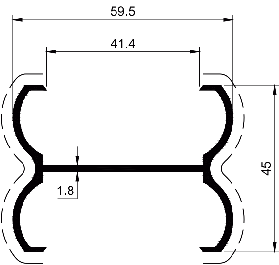
SECTION NO. - HDR-303 EST. WEIGHT - 0.769 KG./M.
