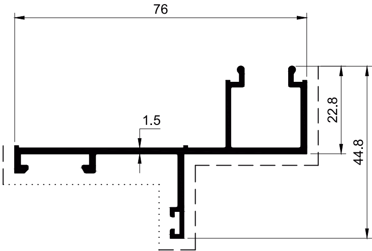
SECTION NO. - PD-108 EST. WEIGHT - 0.649 KG./M.
