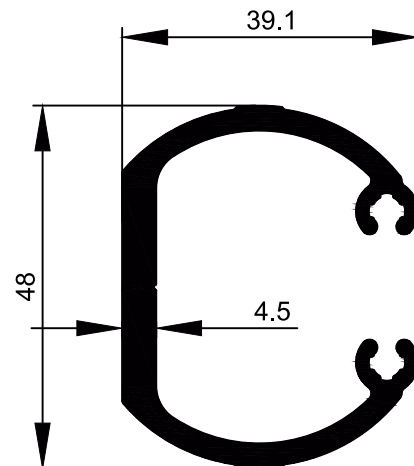
SECTION NO. - CW-509 EST. WEIGHT - 1.165 KG./M.
