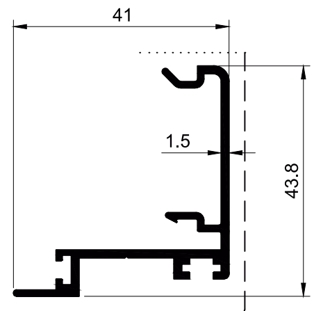
SECTION NO. - ABS-SD15 EST. WEIGHT - 0.490 KG./M.
