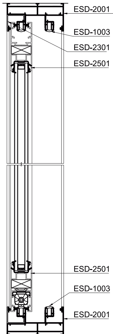
SECTION A-A
