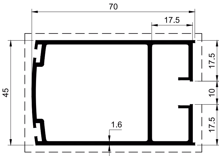
SECTION NO. - 100D - 103 EST. WEIGHT - 1.155 KG./M.
