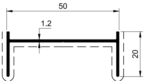
SECTION NO. - SCU-003 EST. WEIGHT - 0.283 KG./M.
