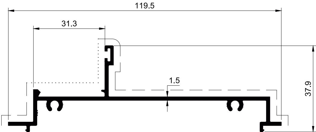
SECTION NO. - 80SFL-1005 EST. WEIGHT - 0.823 KG./M.
