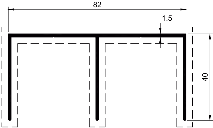
SECTION NO. - ALU-S28 EST. WEIGHT - 0.736 KG./M.
