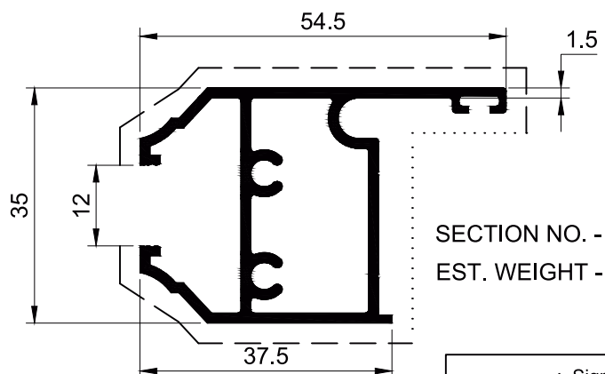
SECTION NO. - CA-1118 EST. WEIGHT - 1.280 KG./M.
