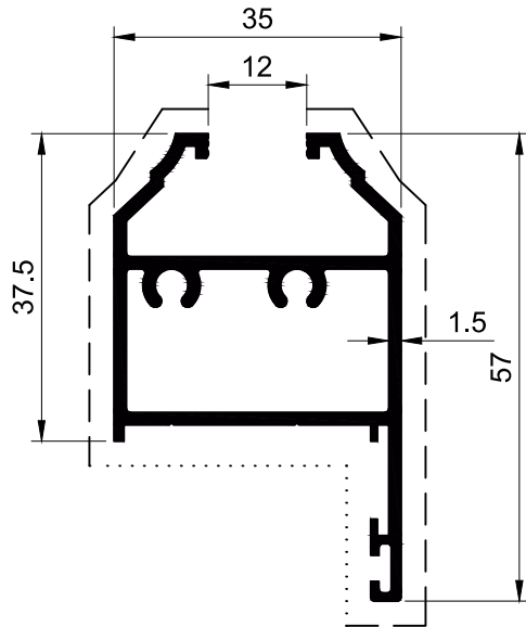
SECTION NO. - CA-2010 EST. WEIGHT - 0.803 KG./M.
