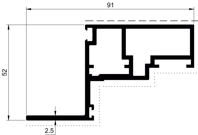
SECTION NO. - CW-514 EST. WEIGHT - 1.603 KG./M.
