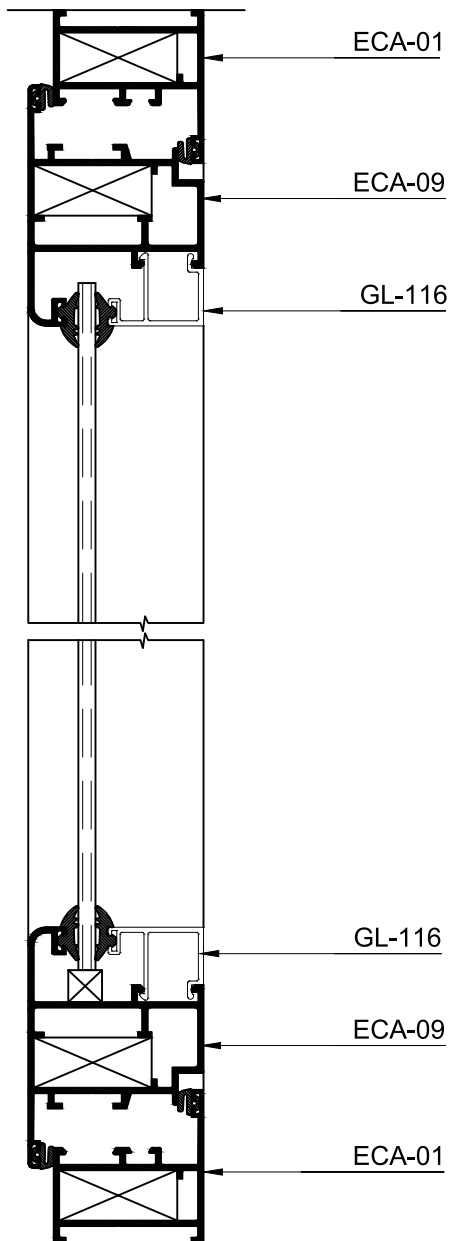
SECTION :- A-A
