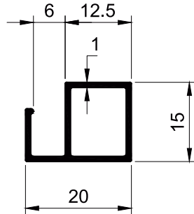
SECTION NO. - KCB-018 EST. WEIGHT - 0.184 KG./M.
