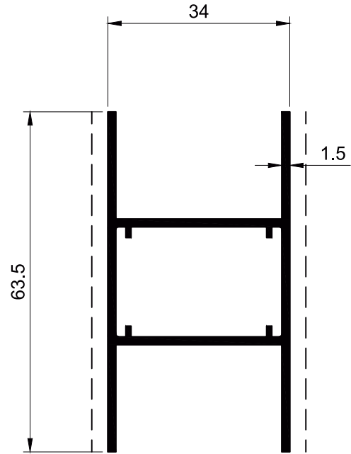
SECTION NO. - PD-110 EST. WEIGHT - 0.788 KG./M.
