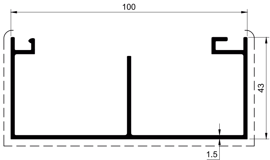
SECTION NO. - HPT-007 EST. WEIGHT - 1.032 KG./M.
