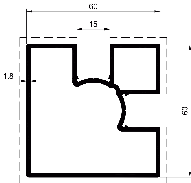
SECTION NO. - HDR-309 EST. WEIGHT - 1.501 KG./M.
