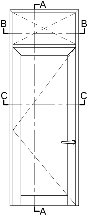
ELEVATION
