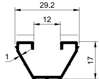
SECTION NO - ESD-2902 EST. WEIGHT - 0.191 KG./M
