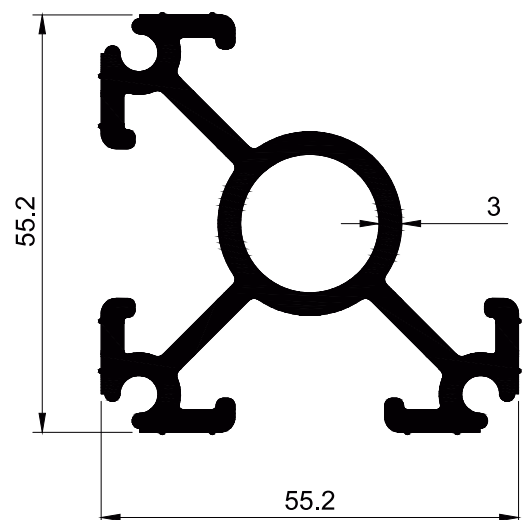
SECTION NO. - HDR-310 EST. WEIGHT - 1.829 KG./M.
