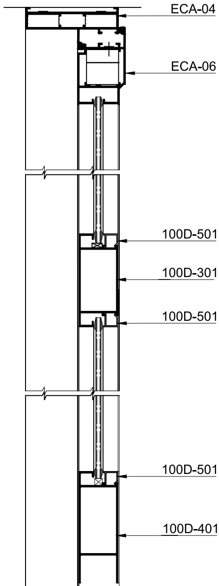
Section :- A-A
