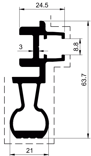
SECTION NO. - ESD-1902 EST. WEIGHT - 1.194 KG./M.
