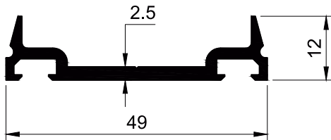
SECTION NO. - CW-506 EST. WEIGHT - 0.422 KG./M.
