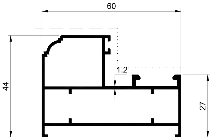
SECTION NO. - PD-201 EST. WEIGHT - 0.756 KG./M.
