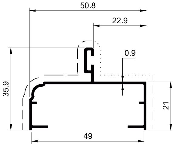
SECTION NO. - WRD-101 EST. WEIGHT - 0.328 KG./M.
