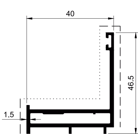
SECTION NO. - CW-510 EST. WEIGHT - 0.583 KG./M.
