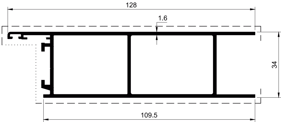
SECTION NO. - PD-102 EST. WEIGHT - 1.485 KG./M.
