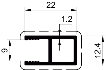
SECTION NO. - SCU-004 EST. WEIGHT - 0.217 KG./M.
