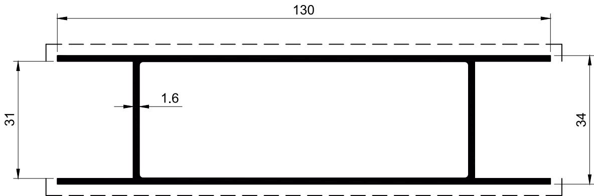
SECTION NO. - PD-103 EST. WEIGHT - 1.370 KG./M.
