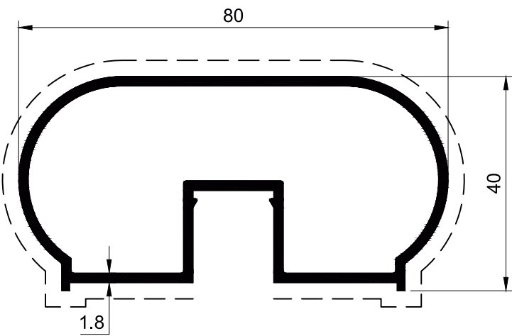
SECTION NO. - HDR-301 EST. WEIGHT - 1.172 KG./M.
