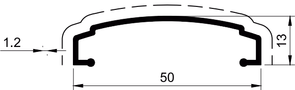
SECTION NO. - HPT-003 EST. WEIGHT - 0.248 KG./M.
