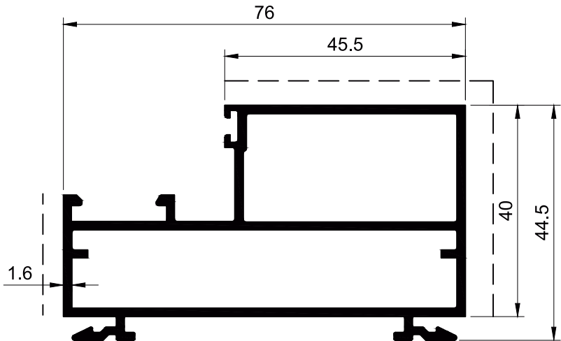
SECTION NO. - PD-101 EST. WEIGHT - 1.370 KG./M.
