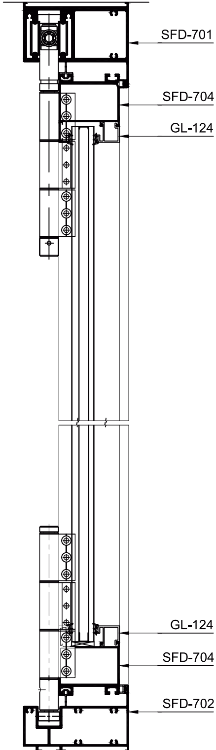
SECTION :- A-A
