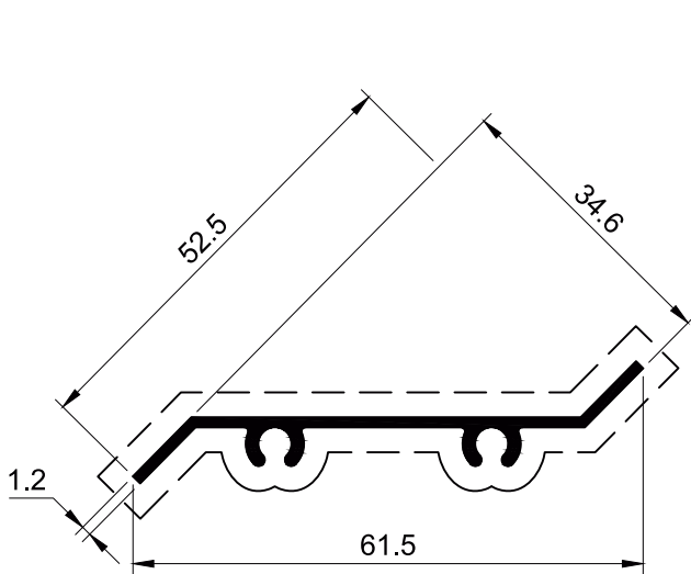
SECTION NO. - DG-01 EST. WEIGHT - 0.298 KG./M.
