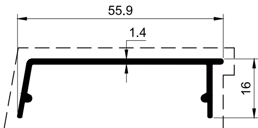
SECTION NO. - CW-508 EST. WEIGHT - 0.322 KG./M.
