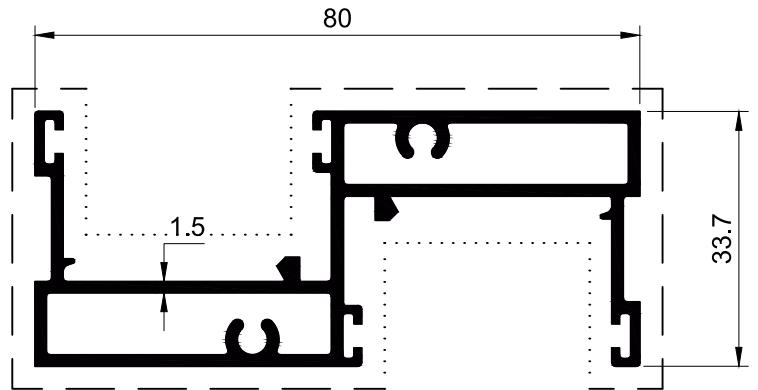
SECTION NO. - 80S-2201 EST. WEIGHT - 1.237 KG./M.
