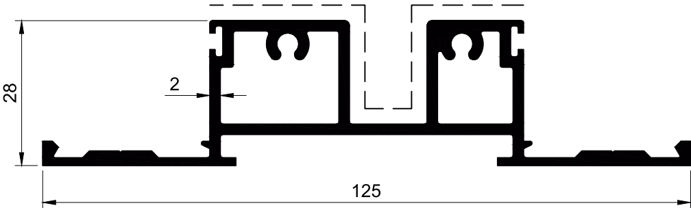
SECTION NO. - SFD-608 EST. WEIGHT - 1.627 KG./M.
