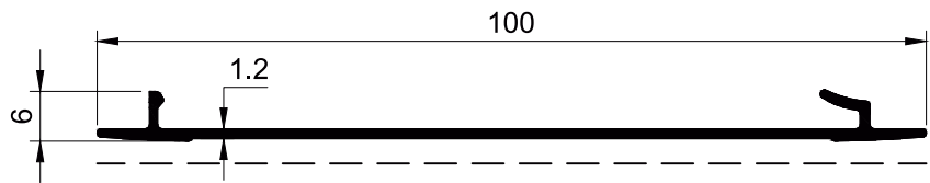
SECTION NO. - HPT-002 EST. WEIGHT - 0.372 KG./M.
