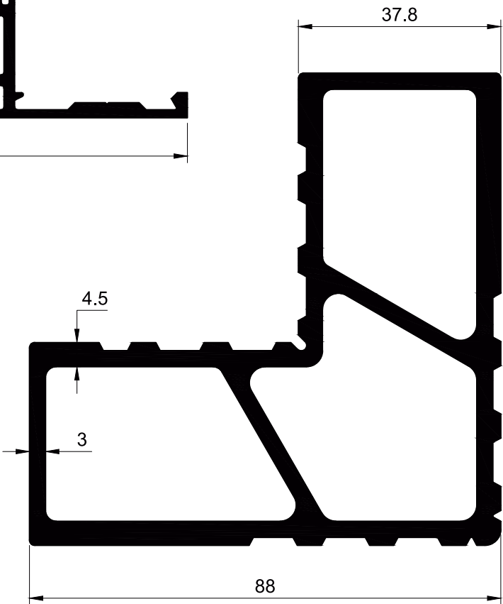
SECTION NO. - SFD-606 EST. WEIGHT - 4.040 KG./M.
