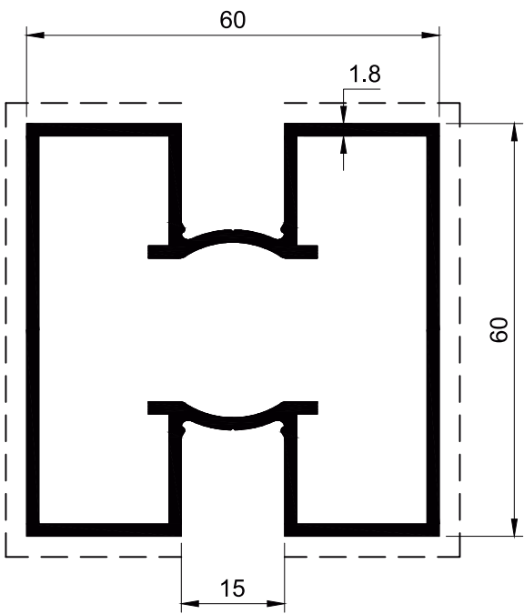
SECTION NO. - HDR-302 EST. WEIGHT - 1.555 KG./M.
