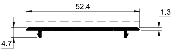
SECTION NO. - HDR-306 EST. WEIGHT - 0.228 KG./M.
