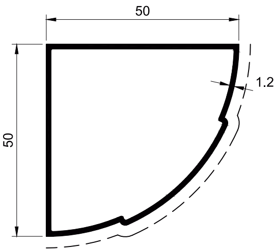
SECTION NO. - HPT-005 EST. WEIGHT - 0.575 KG./M.
