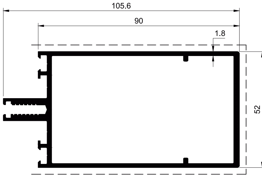
SECTION NO. - CW-505 EST. WEIGHT - 1.809 KG./M.
