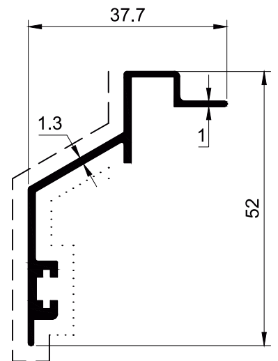
SECTION NO. - ABS-SD11 EST. WEIGHT - 0.359 KG./M.
