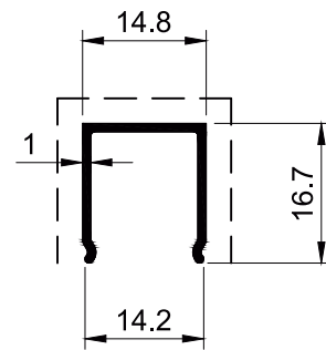
SECTION NO. - HDR-307 EST. WEIGHT - 0.125 KG./M.
